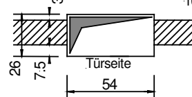
Grundriss Aussparung
