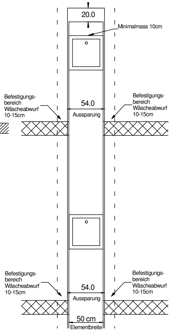
Grundriss Aussparung
