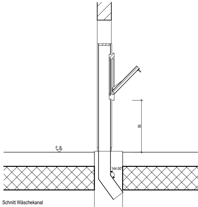
Schnitt Wäschekanal
