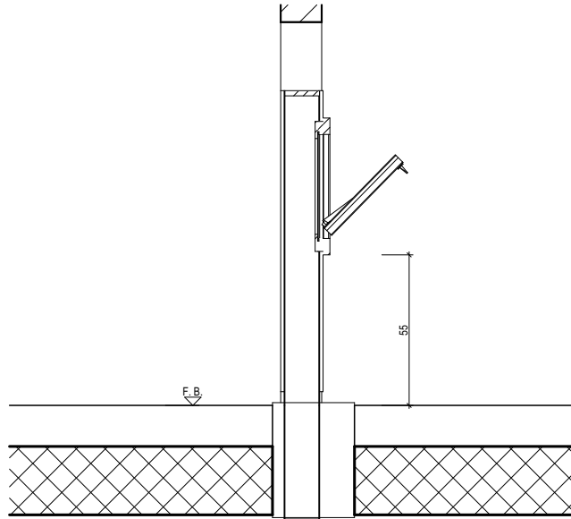
Schnitt Wäschekanal
