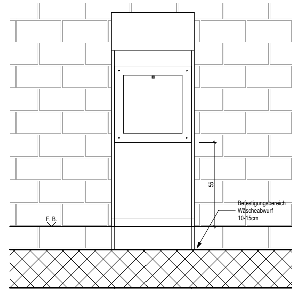
Frontansicht
