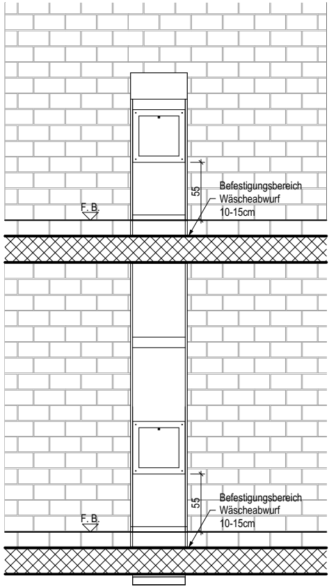
Frontansicht
