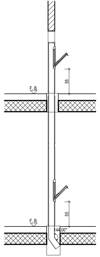
Schnitt Wäschekanal
