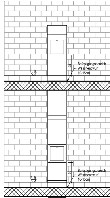
Frontansicht
