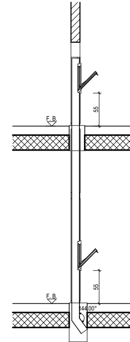
Schnitt Wäschekanal
