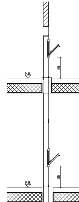
Schnitt Wäschekanal
